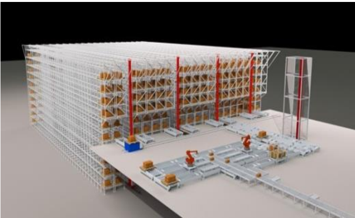
双深位自动化仓库
